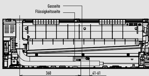
Rückansicht
