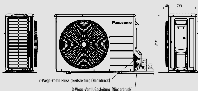
Seitenansicht
