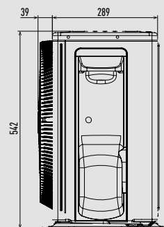
Seitenansicht
