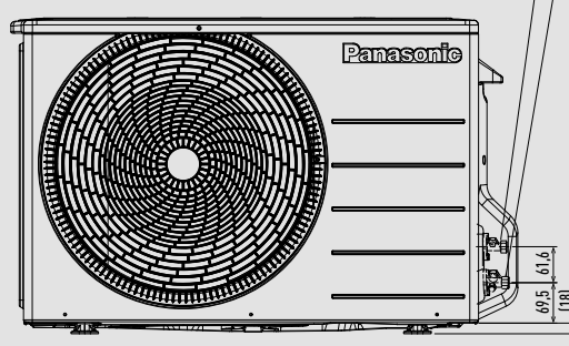
Frontansicht
