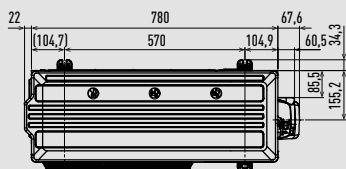
Frontansicht
