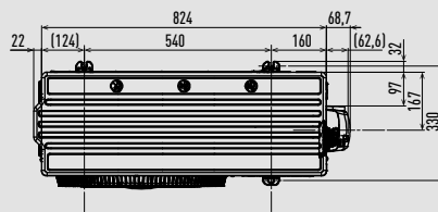
Frontansicht
