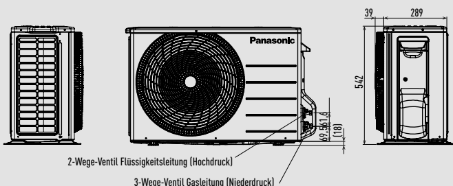
Seitenansicht
