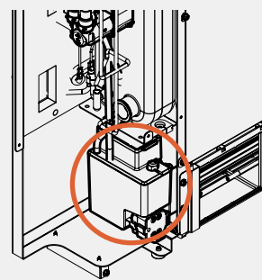
Einspritz-Set
