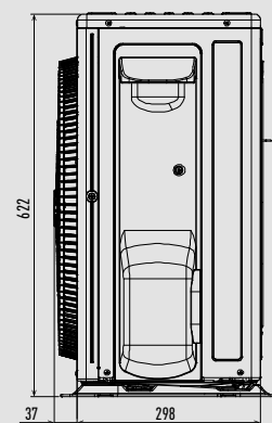
Seitenansicht
